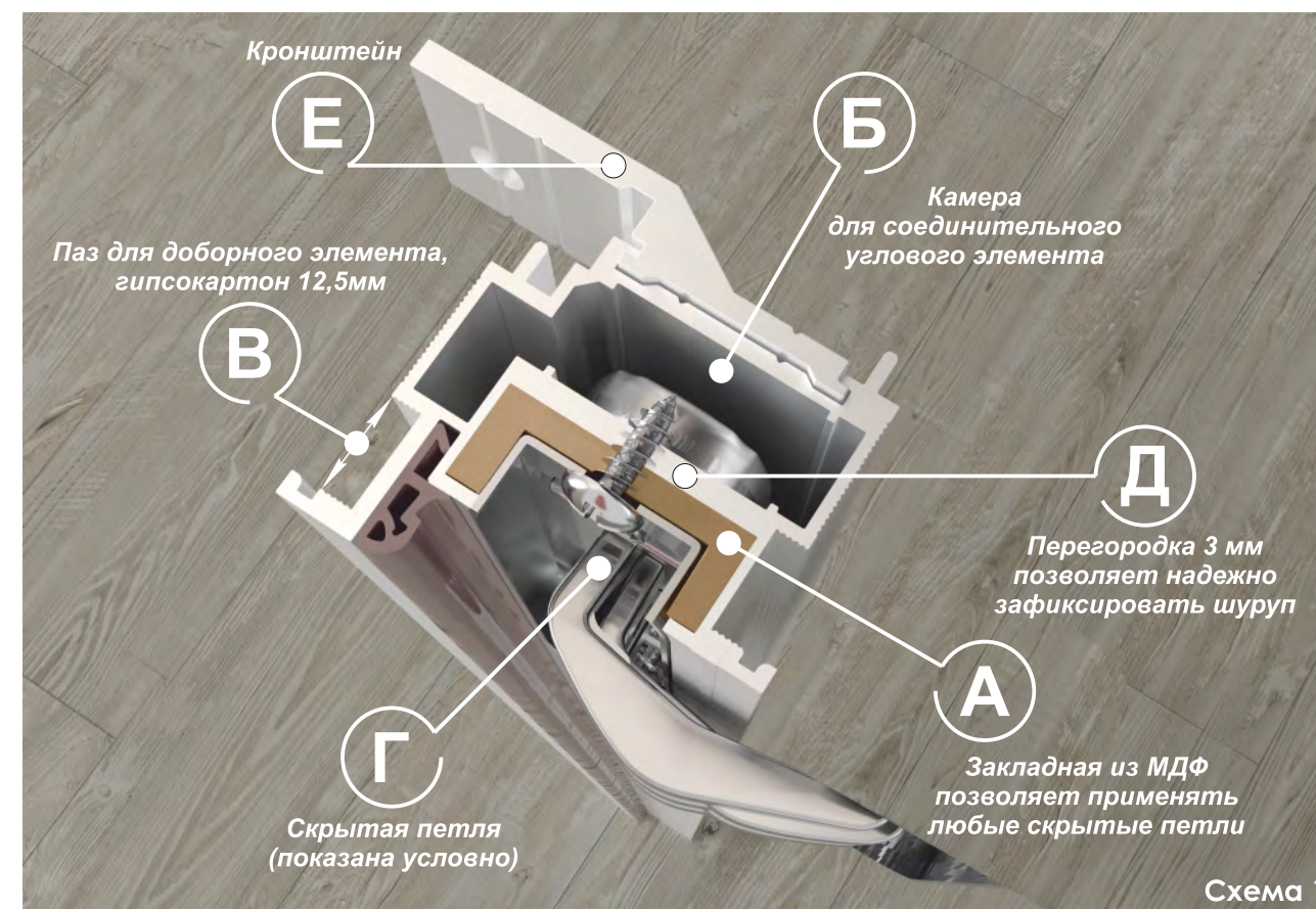
Схема фиксации угловых соединений в бруске коробочном БК-33
